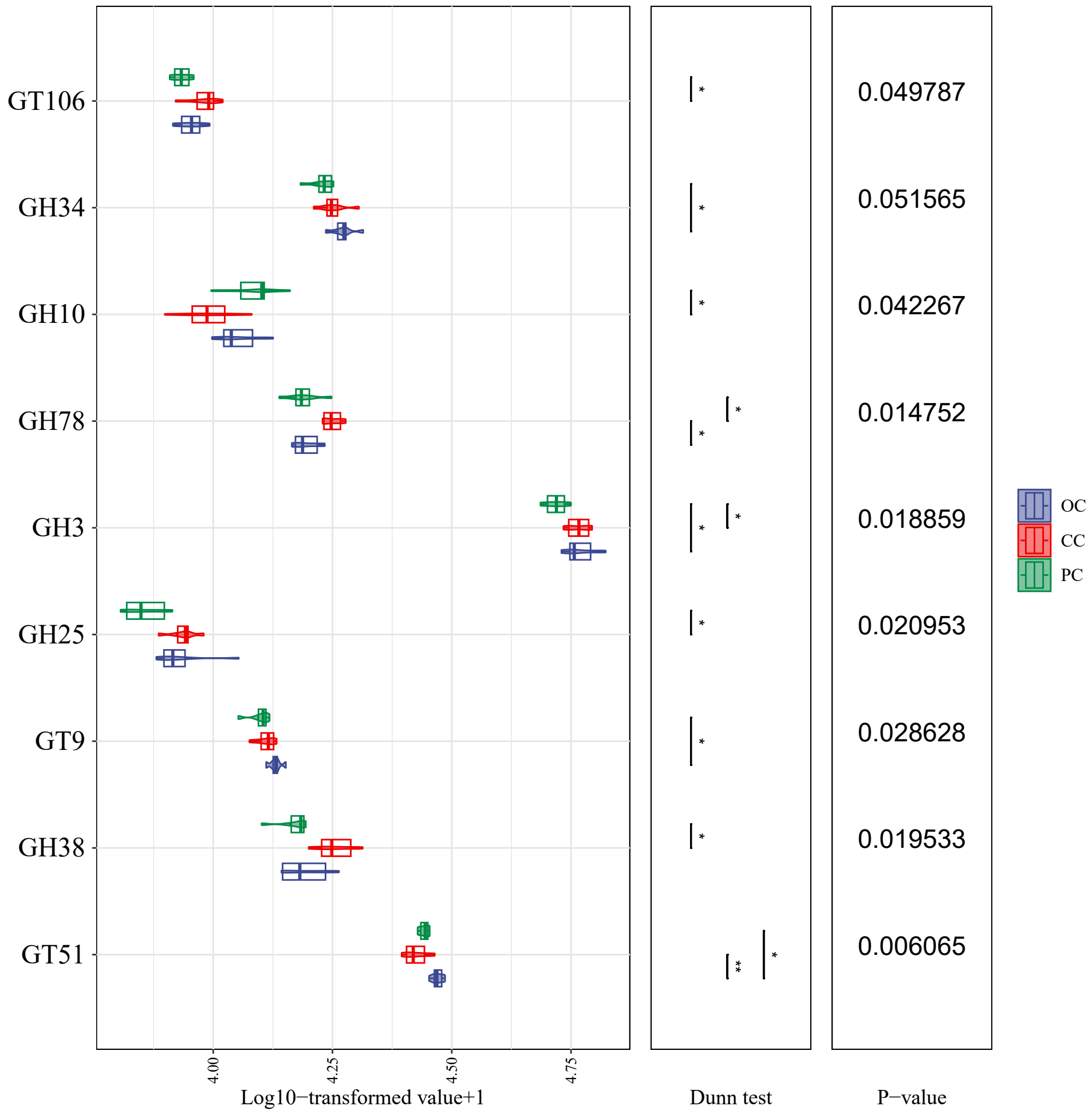
Kruskal–Wallis test
